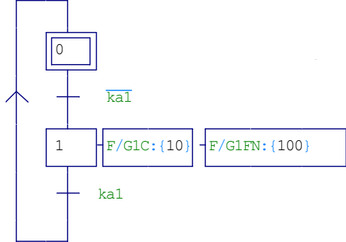
G1S : GRAFCET de sécurité de la station 1
