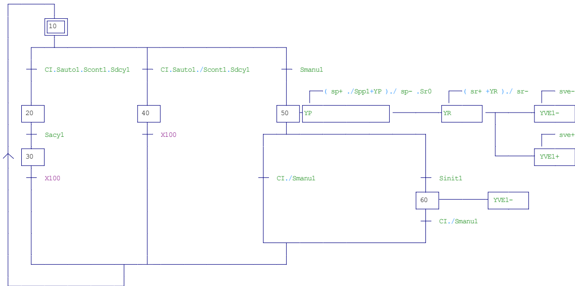
G1FN : GRAFCET de Fonctionnement Normal de la station 1
