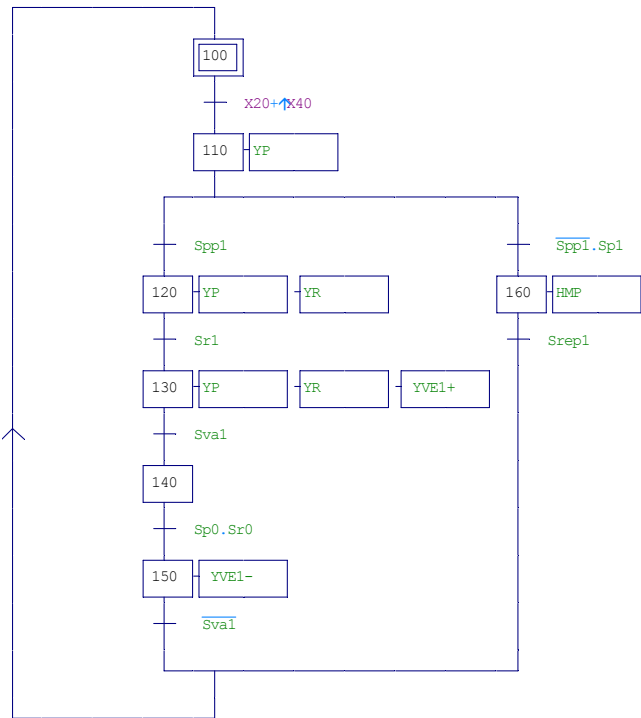
G1FN : GRAFCET de Fonctionnement Normal de la station 1
